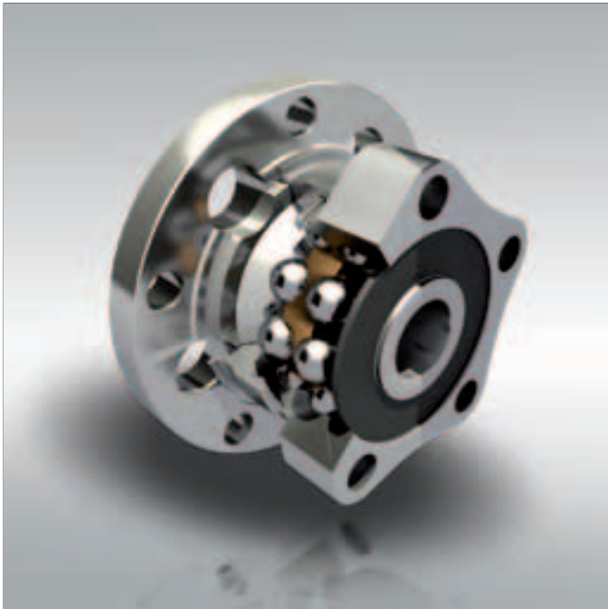
Rys. 9 Piasta trzeciej generacji
