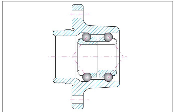
Rys. 8 Piasta drugiej generacji
