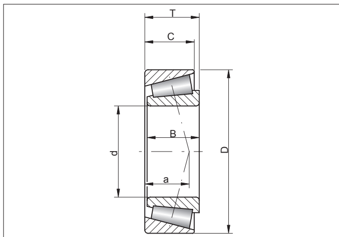
Rys. 3 Łożysko stożkowe jednorzędowe
