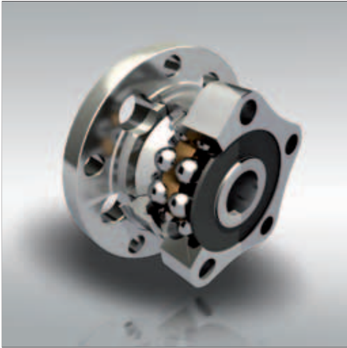
Рис. 9 Ступица третьего поколения
