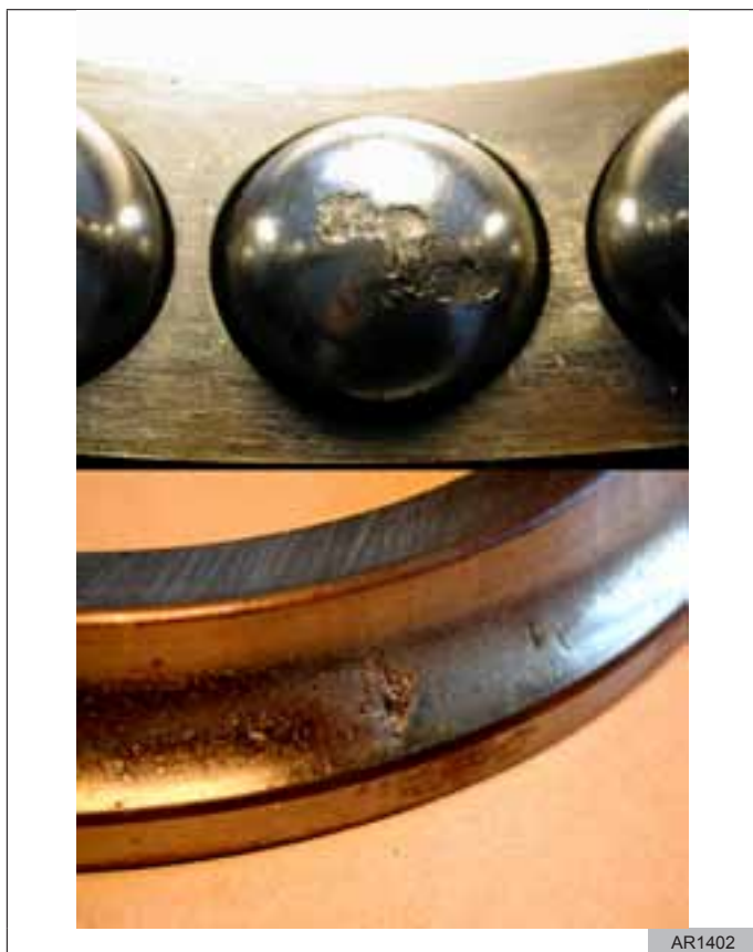
Рис. 30 Видимый износ материалов компонента подшипника
