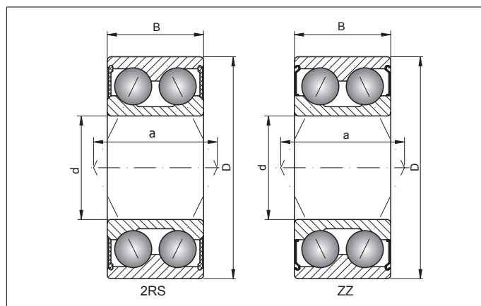
Rys. 4 Łożysko kulkowe skośne dwurzędowe
