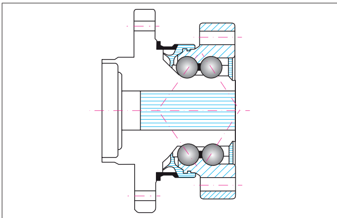
Rys. 10 Piasta trzeciej generacji
