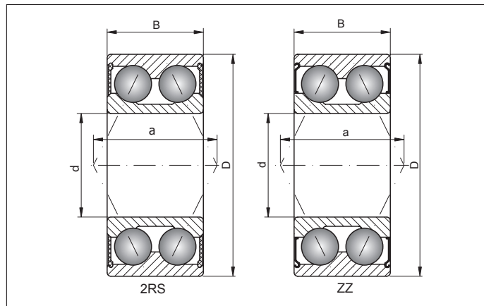
Рис. 4 Двухрядный радиально-упорный подшипник
